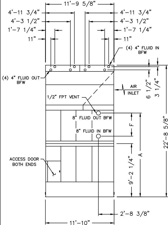
END ELEVATION
