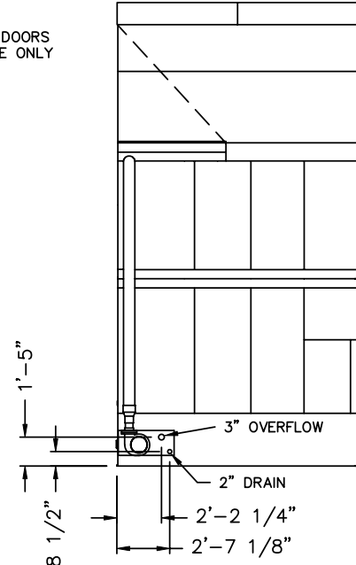
END ELEVATION
