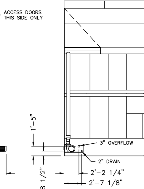
END ELEVATION
